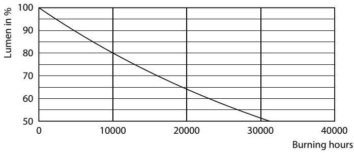
LEDBulb E26
